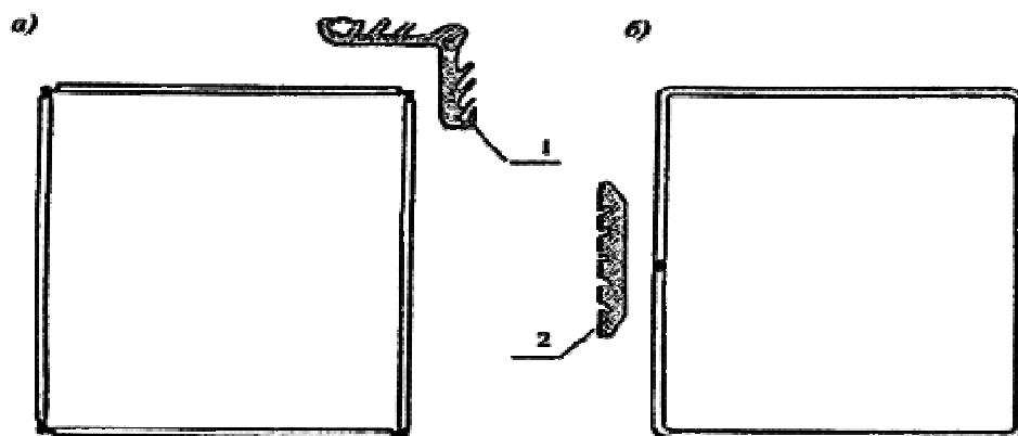
а - дистанционная рамка из прямолинейных деталей, собранная на четырех соединительных уголках (1); б - дистанционная рамка, изготовленная методом гнутья и замкнутая на одном соединителе (2)
