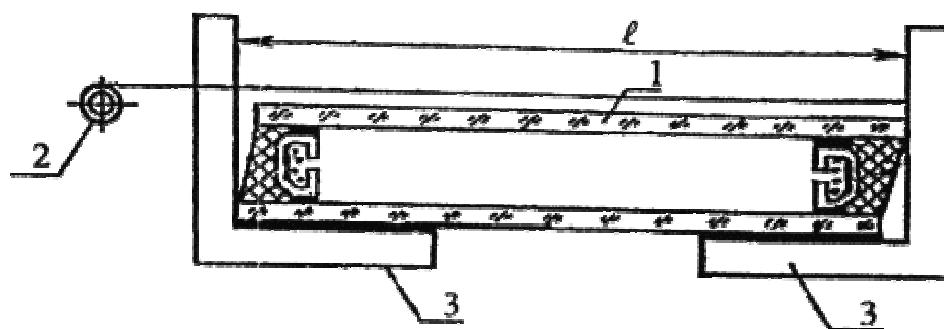
1 - стеклопакет; 2 - рулетка; 3 - угольник; l - контролируемый размер
